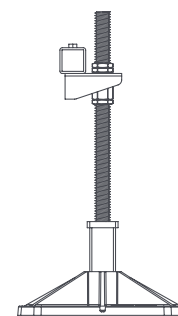
Lange schroefpoot Hoogte-instelling: 335 - 660 mm
