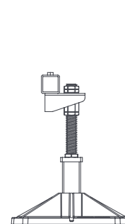
Standaard poot Hoogte-instelling: 335 - 440 mm
